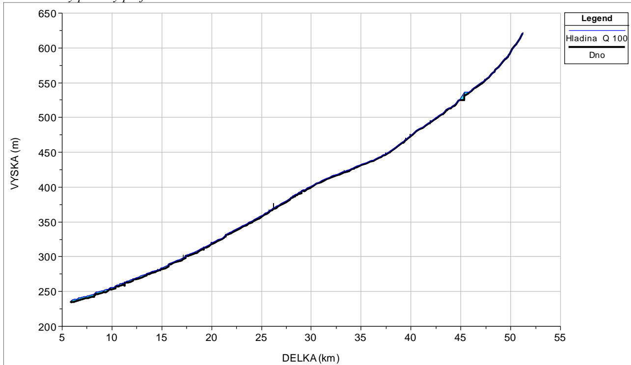
Přehledný podélný profil
